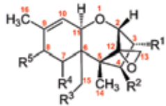
Trichothecenes
