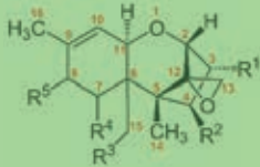
Trichothecenes
