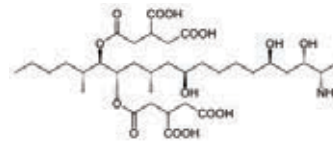
Fumonisin
