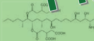
Fumonisin
